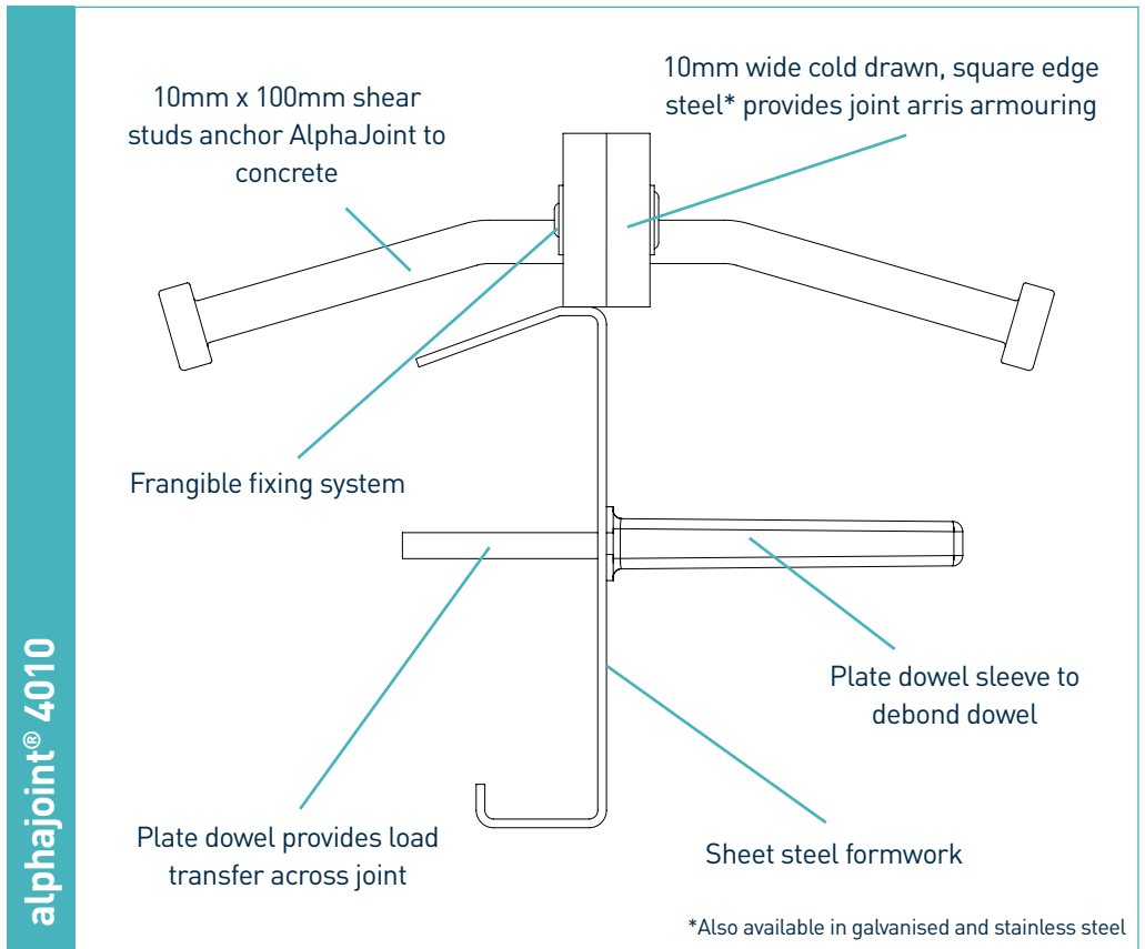
alphajoint® 4010
