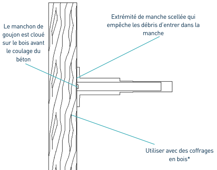
Système de cheville à plaque illustré.
