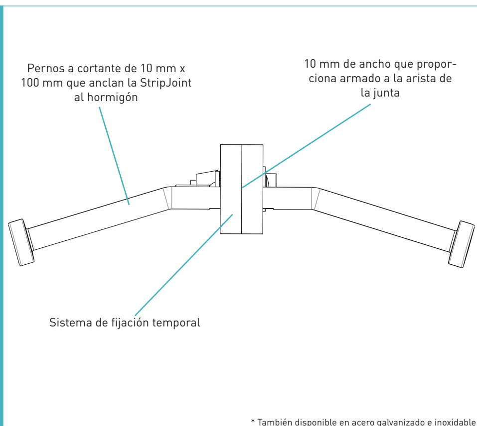
StripJoint Double
