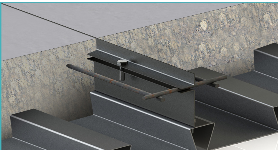
Permadeck Type 1® Pico
